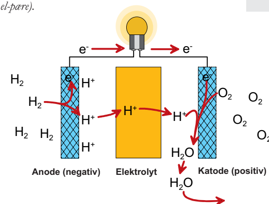
Figur 1. Principskitse for reaktioner og massestrømme i en brændselscelle med en protonledende elektrolyt. Fra venstre kommer H 2 ind, oxideres til H + (afgiver elektroner til elektroden), transporteres gennem elektrolytten og reagerer med O 2 , der samtidig modtager elektroner fra elektroden. Reaktionsproduktet er vand. Elektronerne bevæger sig i det ydre elektriske kredsløb, hvor den elektriske energi afleveres (her i en el-pære).
